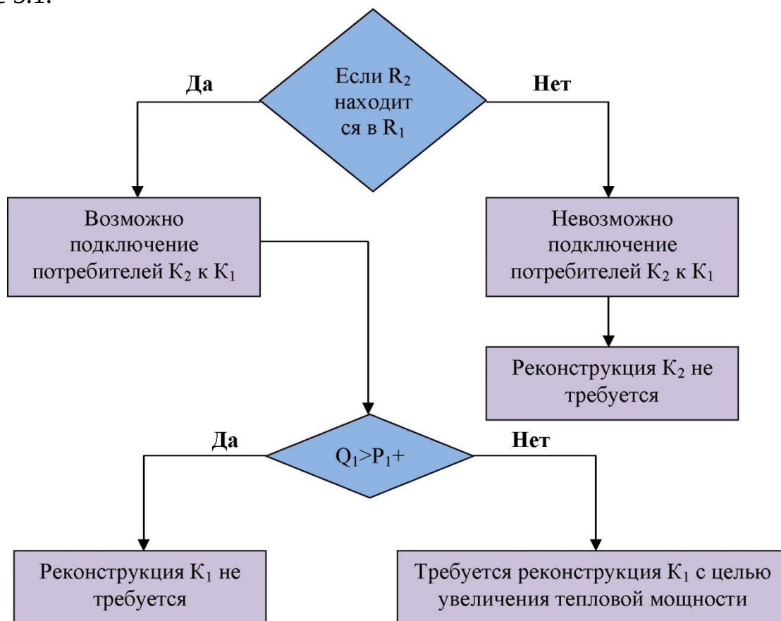
Рисунок 5.1 - Блок-схема обоснования реконструкции котельной K 2 , K 2 - котельная №1 и котельная №2;
